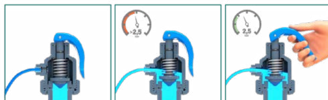
Apertura automatica Automatic opening
