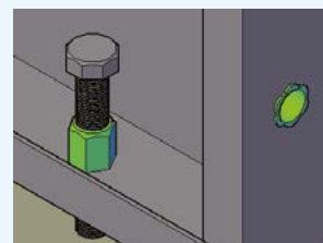
Vite di regolazione su inserto filettato per messa a livello pannello (PLUS)
