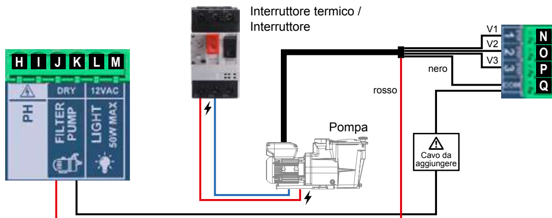
Schema di installazione di una pompa a velocità variabile su AquaRite® UV LS
